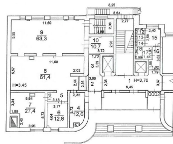
ПЛАН 1 ЭТАЖА
